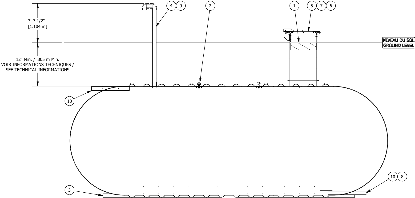
VUE D'ÉLEVATION COUPÉE CUT ELEVATION VIEW
