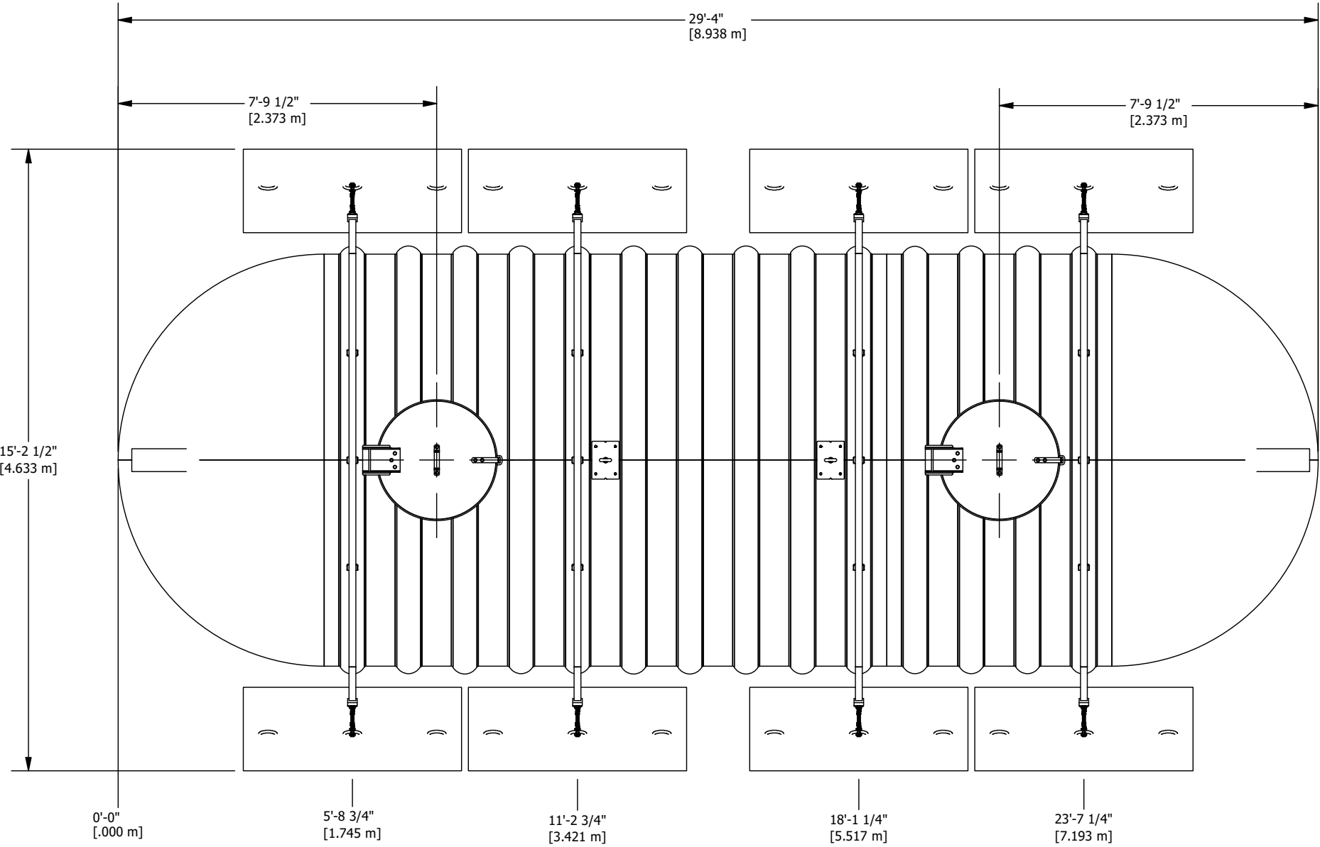
VUE DE PLAN PLAN VIEW
