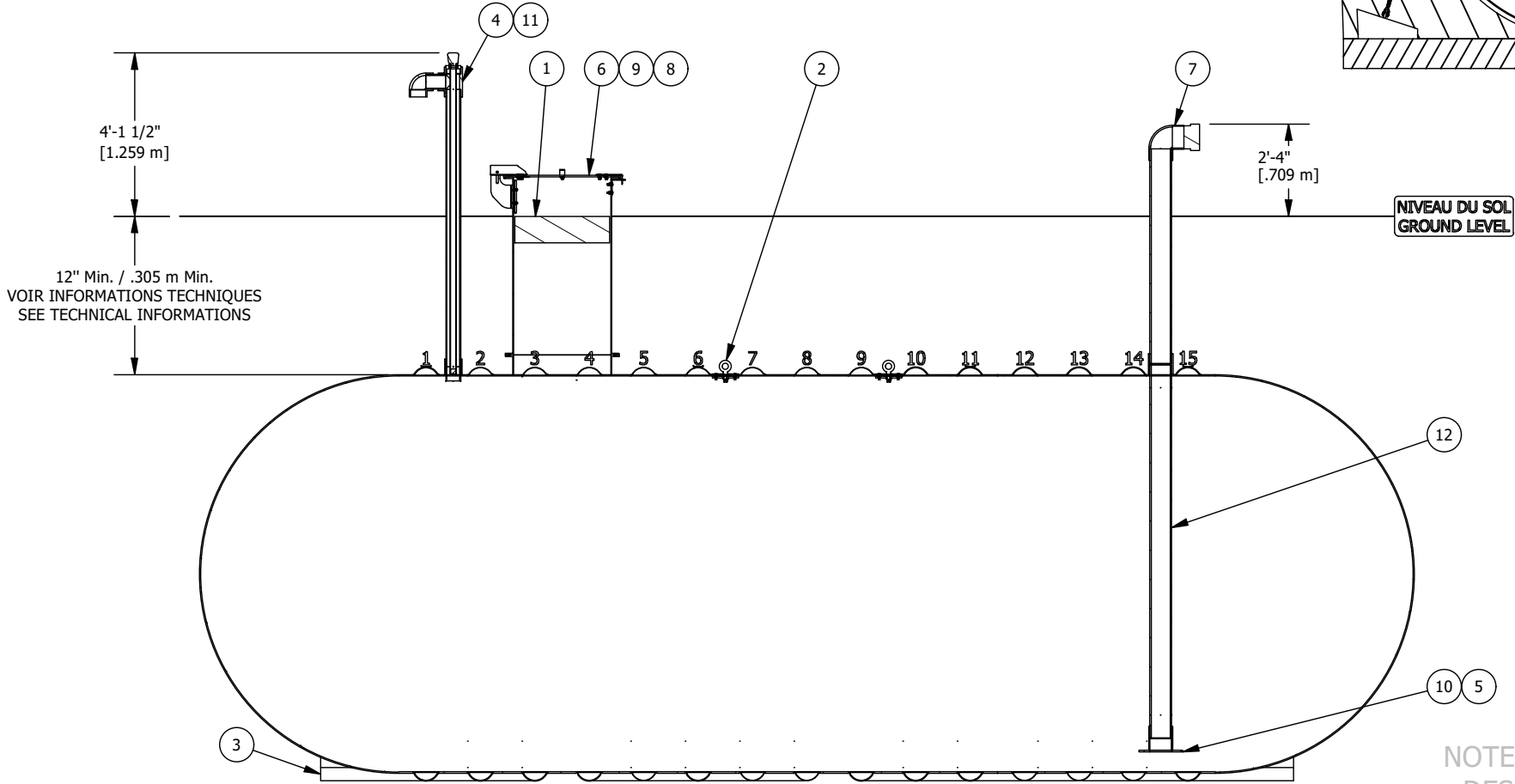
VUE D'ÉLEVATION COUPÉE CUT ELEVATION VIEW
