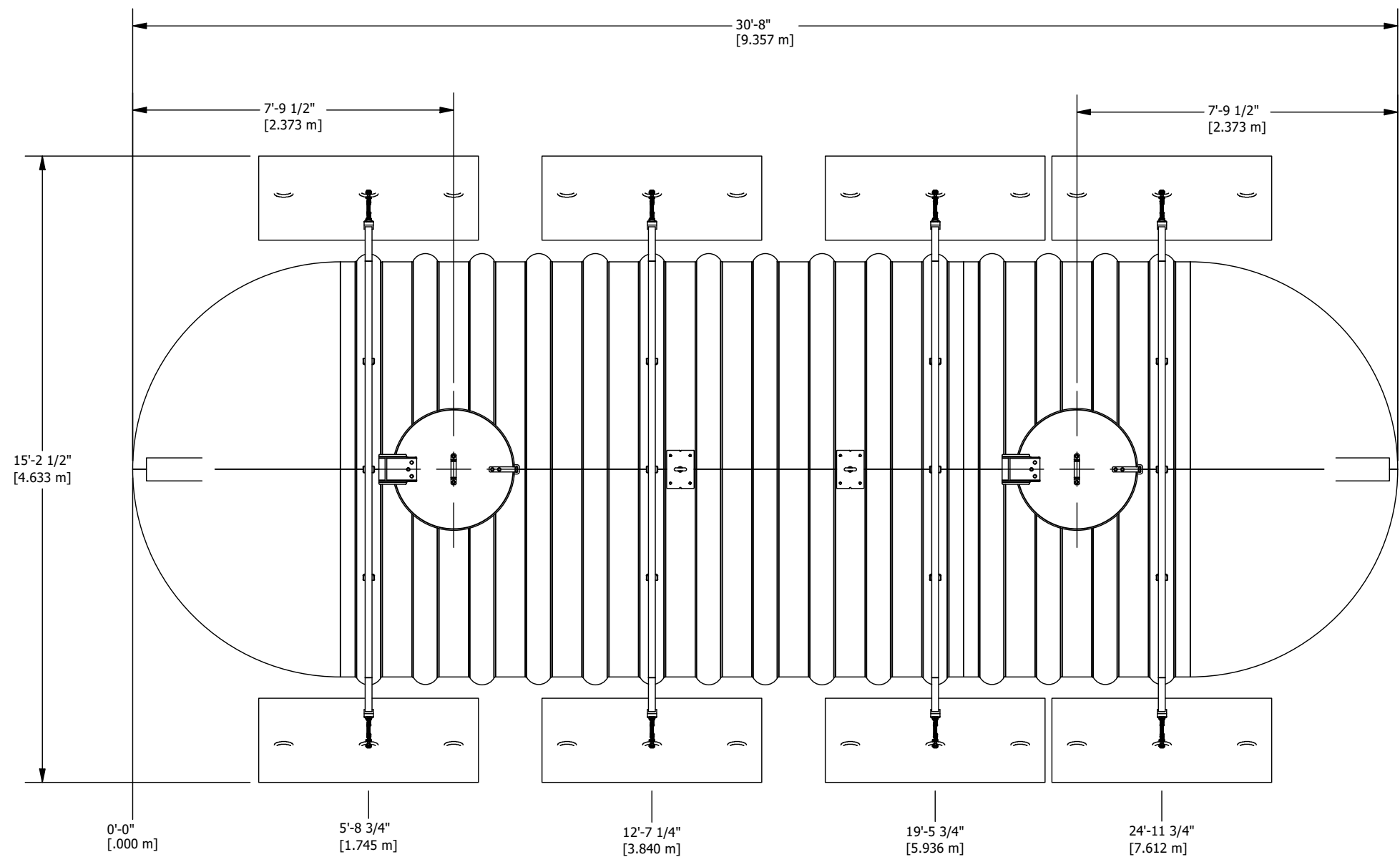
VUE DE PLAN PLAN VIEW
