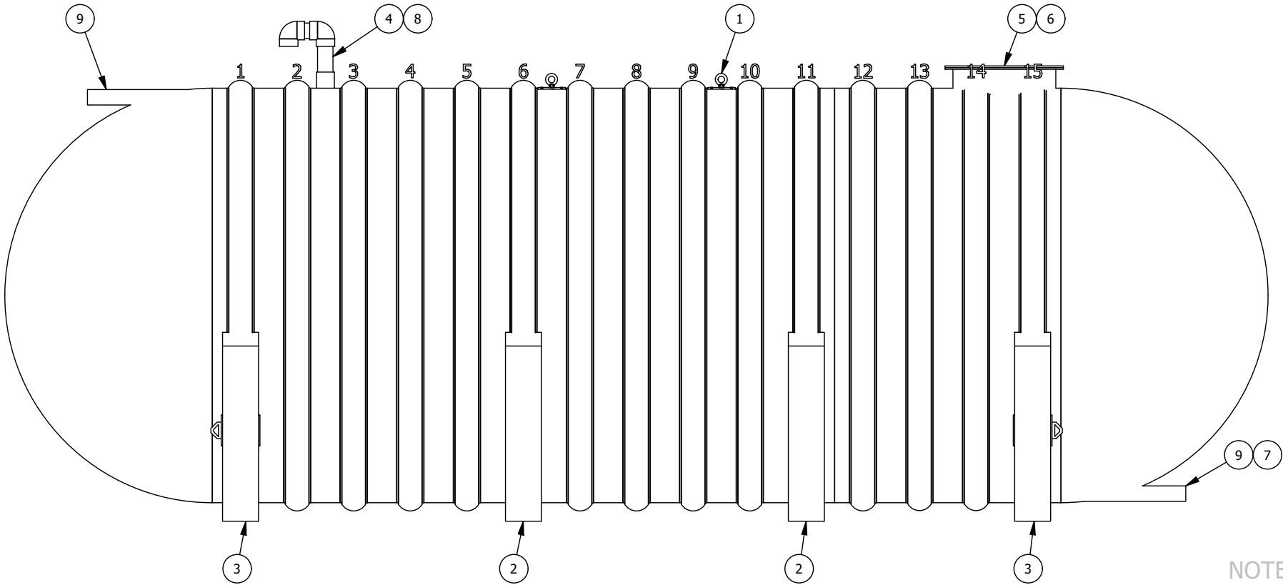
VUE D'ÉLÉVATION ELEVATION VIEW
