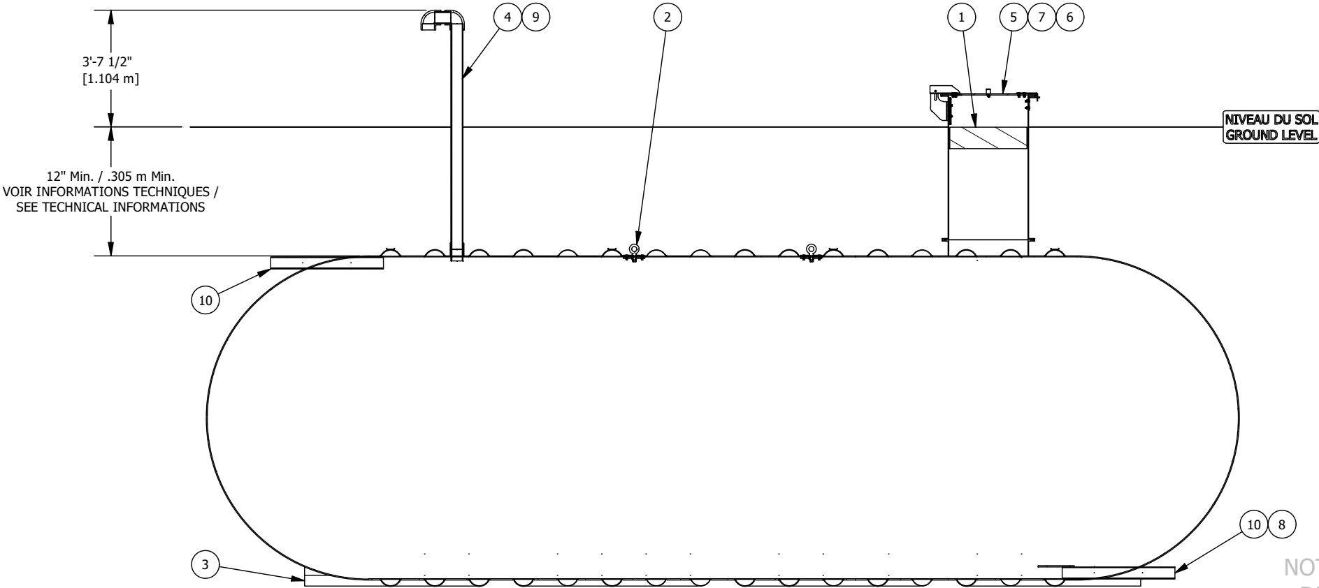
VUE D'ÉLEVATION COUPÉE CUT ELEVATION VIEW
