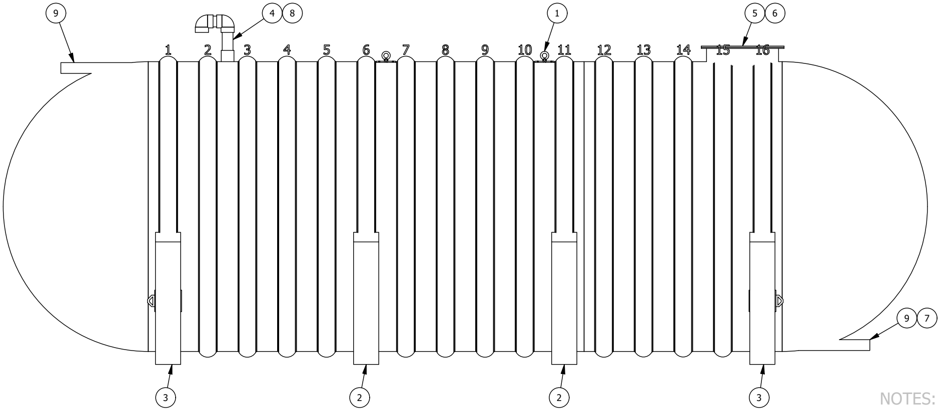
VUE D'ÉLÉVATION ELEVATION VIEW
