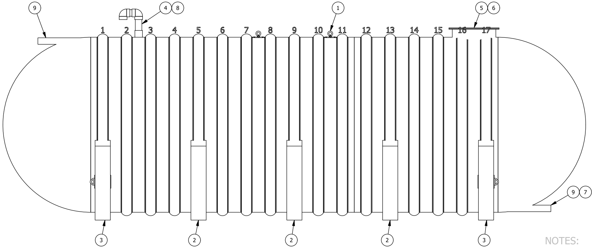
VUE D'ÉLÉVATION ELEVATION VIEW
