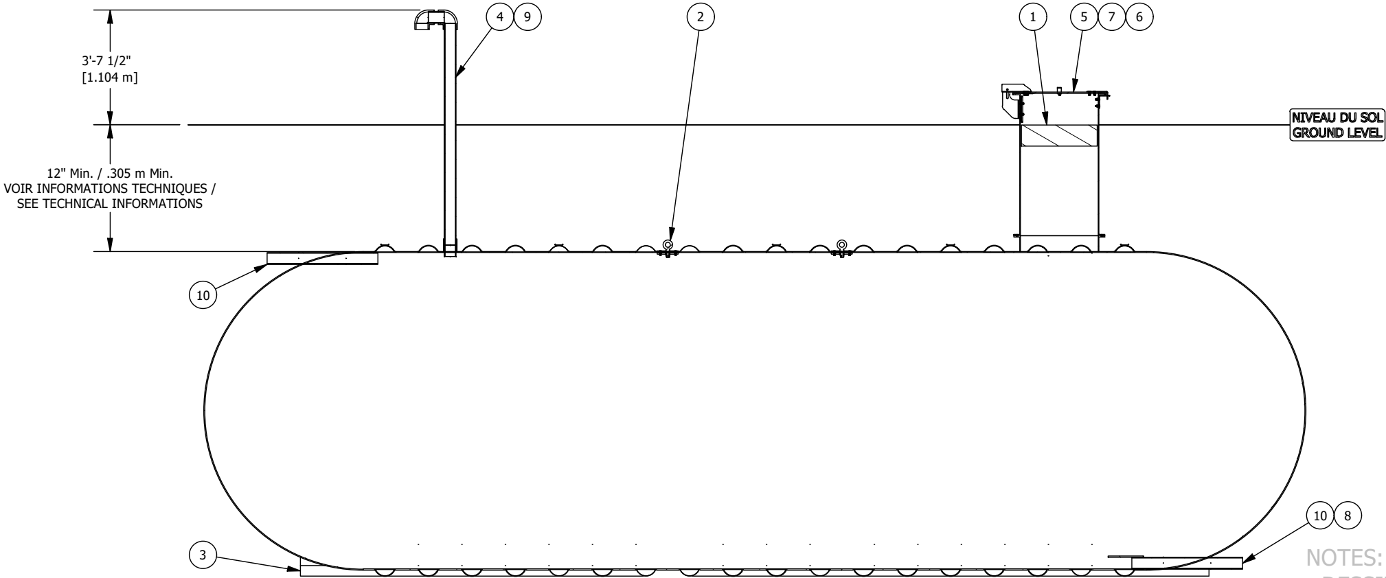
VUE D'ÉLEVATION COUPÉE CUT ELEVATION VIEW
