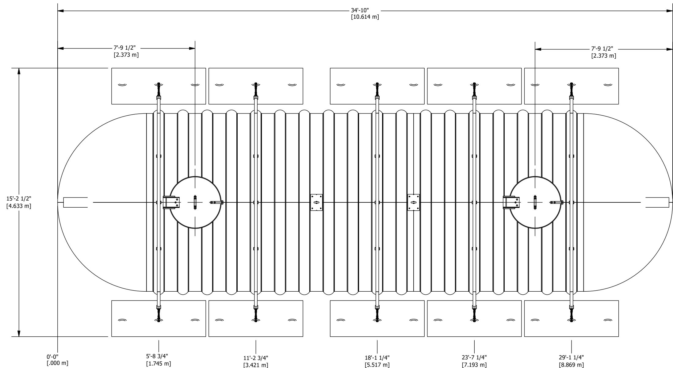
VUE DE PLAN PLAN VIEW
