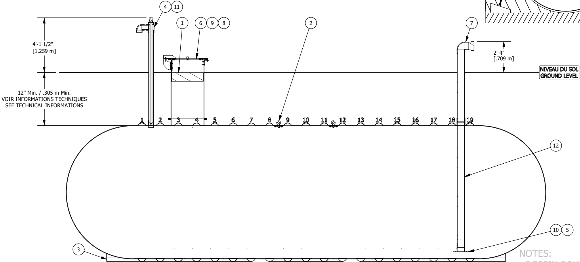
VUE D'ÉLÉVATION COUPÉE CUT ELEVATION VIEW
