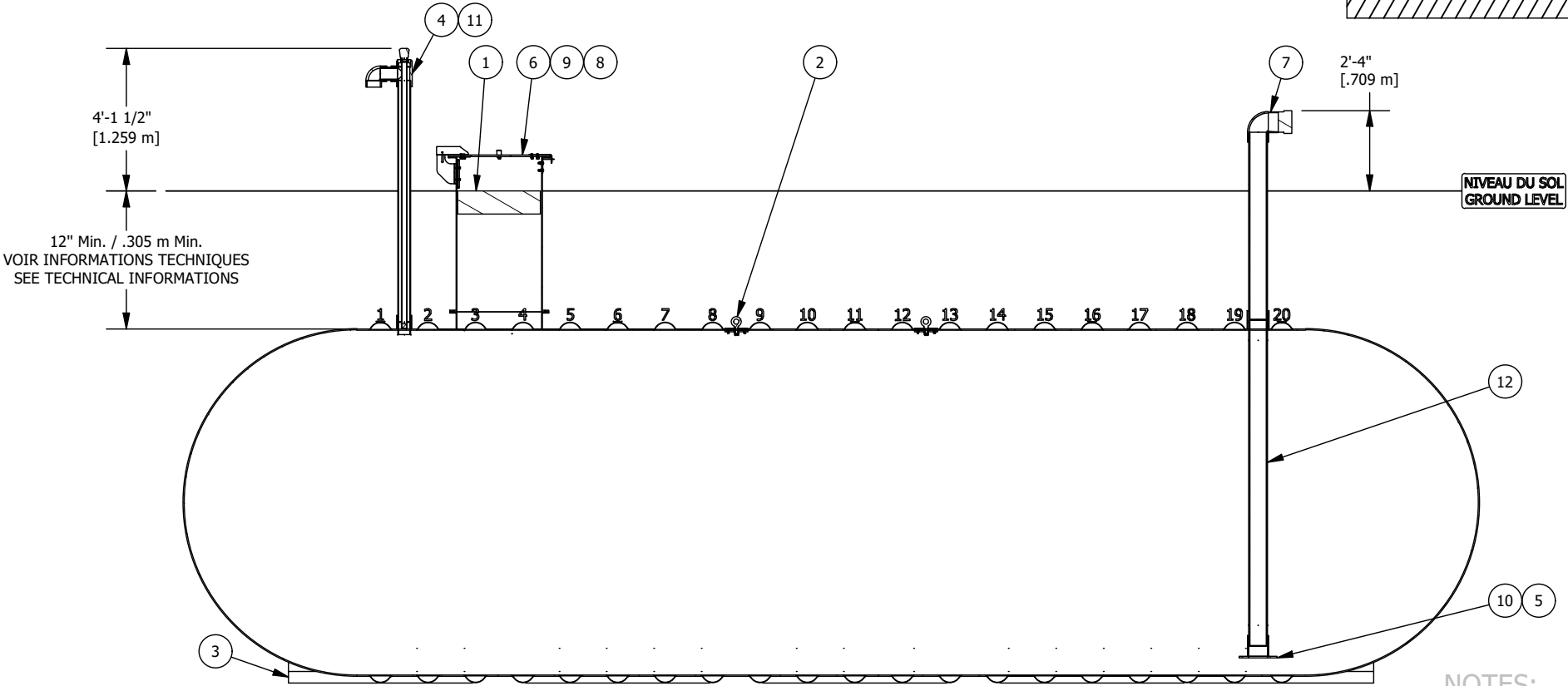
VUE D'ÉLEVATION COUPÉE CUT ELEVATION VIEW
