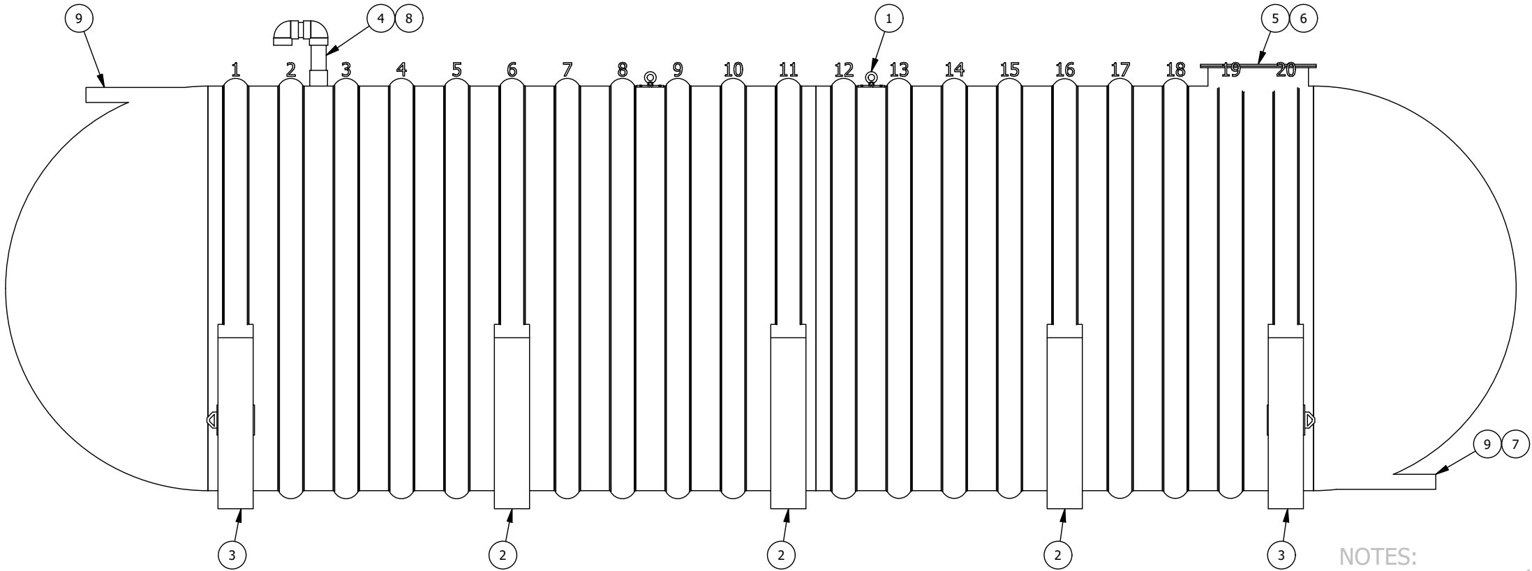
VUE D'ÉLEVATION ELEVATION VIEW
