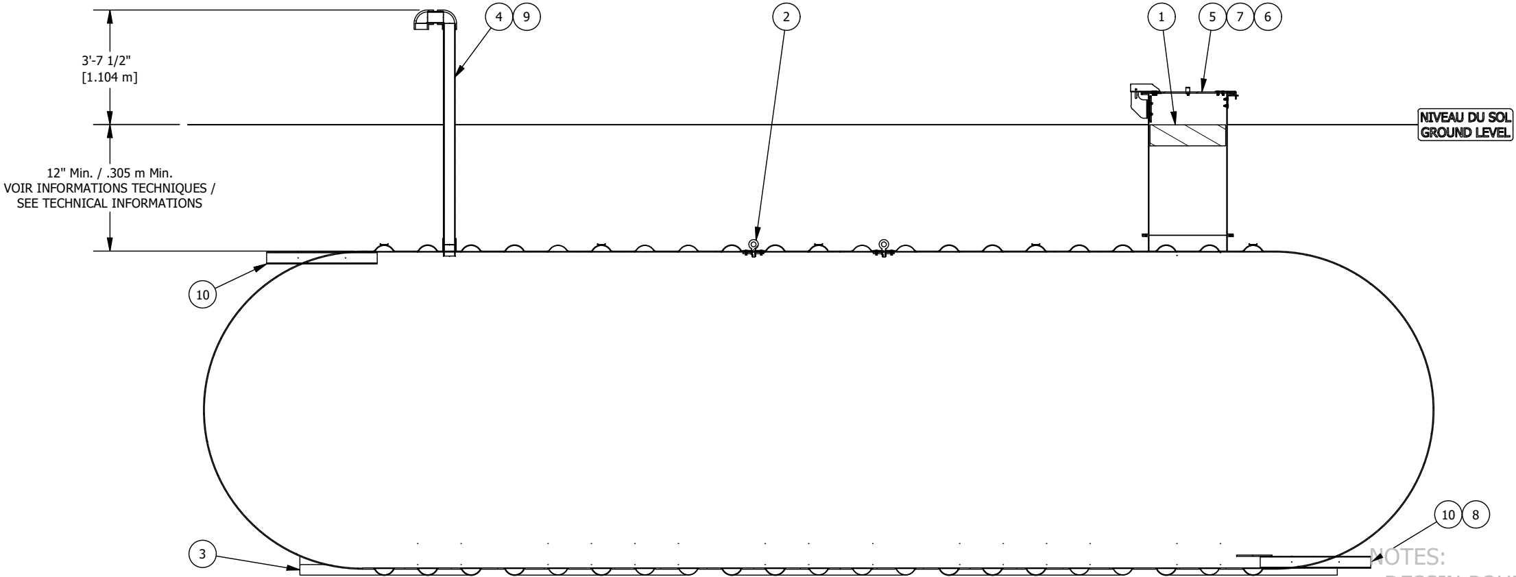
VUE D'ÉLEVATION COUPÉE CUT ELEVATION VIEW
