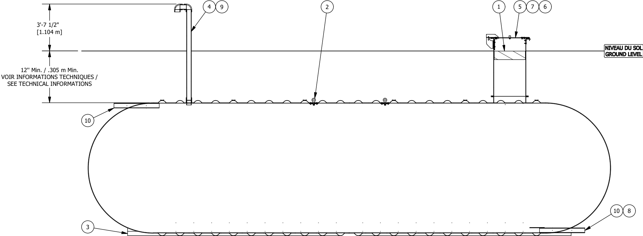
VUE D'ÉLEVATION COUPÉE CUT ELEVATION VIEW
