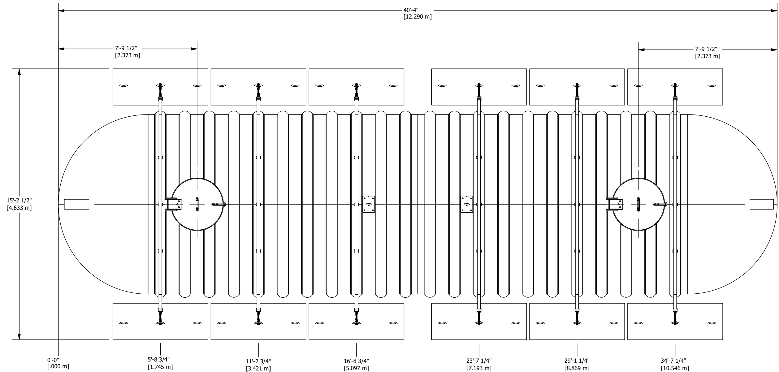
VUE DE PLAN PLAN VIEW
