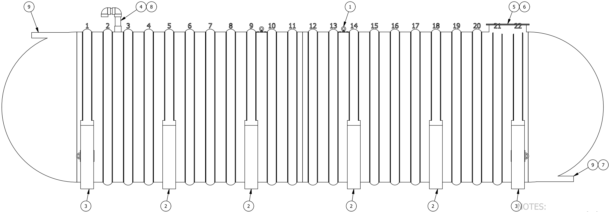
VUE D'ÉLÉVATION ELEVATION VIEW
