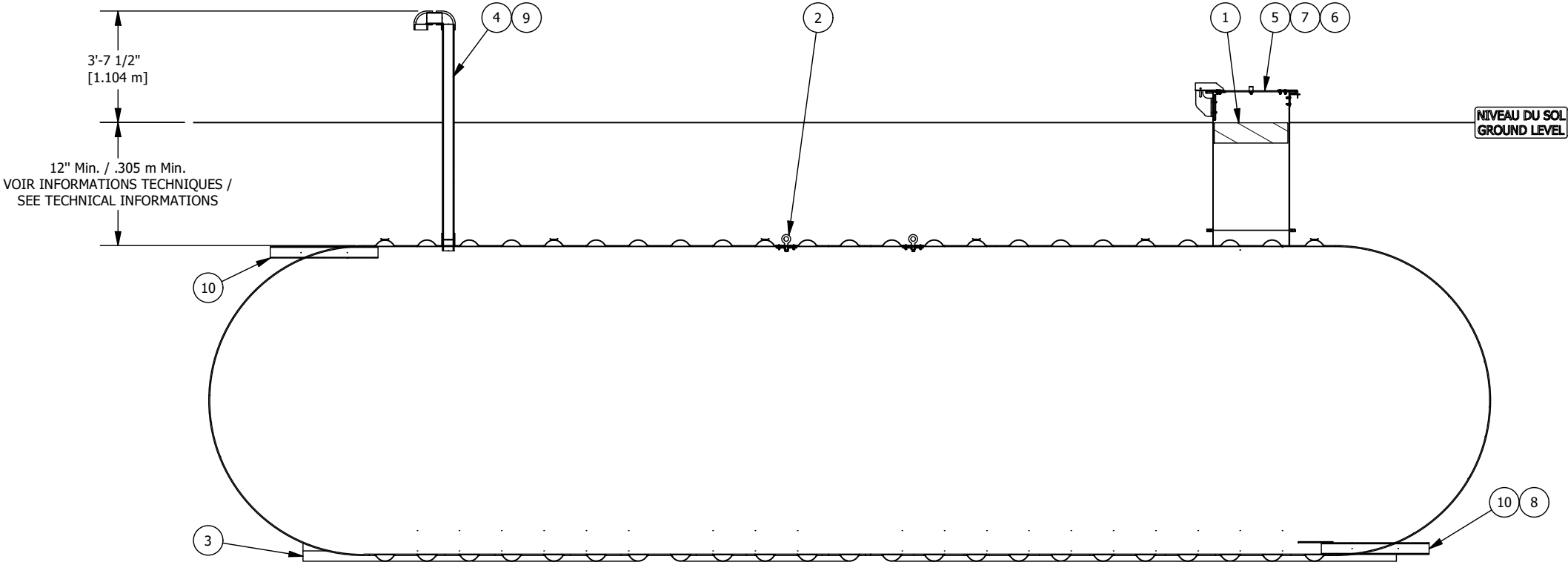
VUE D'ÉLEVATION COUPÉE CUT ELEVATION VIEW
