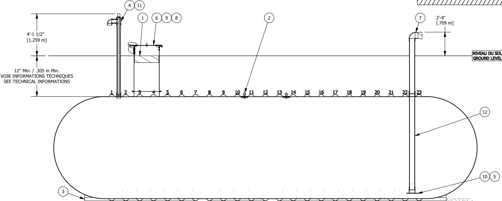
VUE D'ÉLEVATION COUPÉE CUT ELEVATION VIEW
