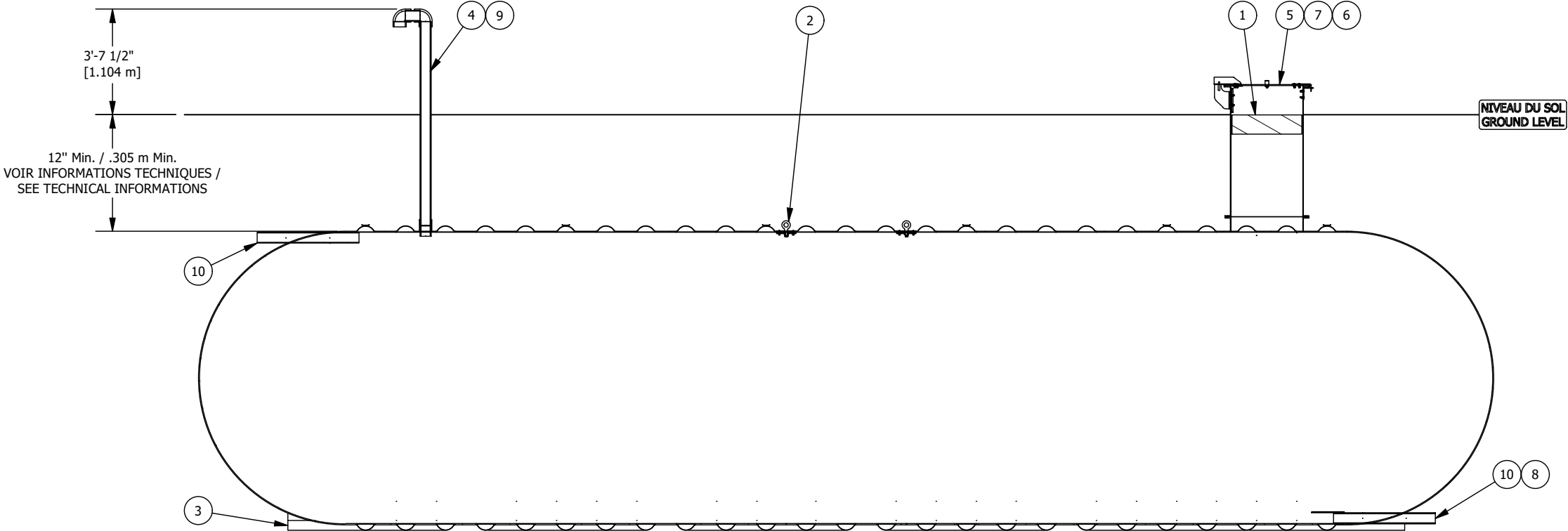
VUE D'ÉLEVATION COUPÉE CUT ELEVATION VIEW
