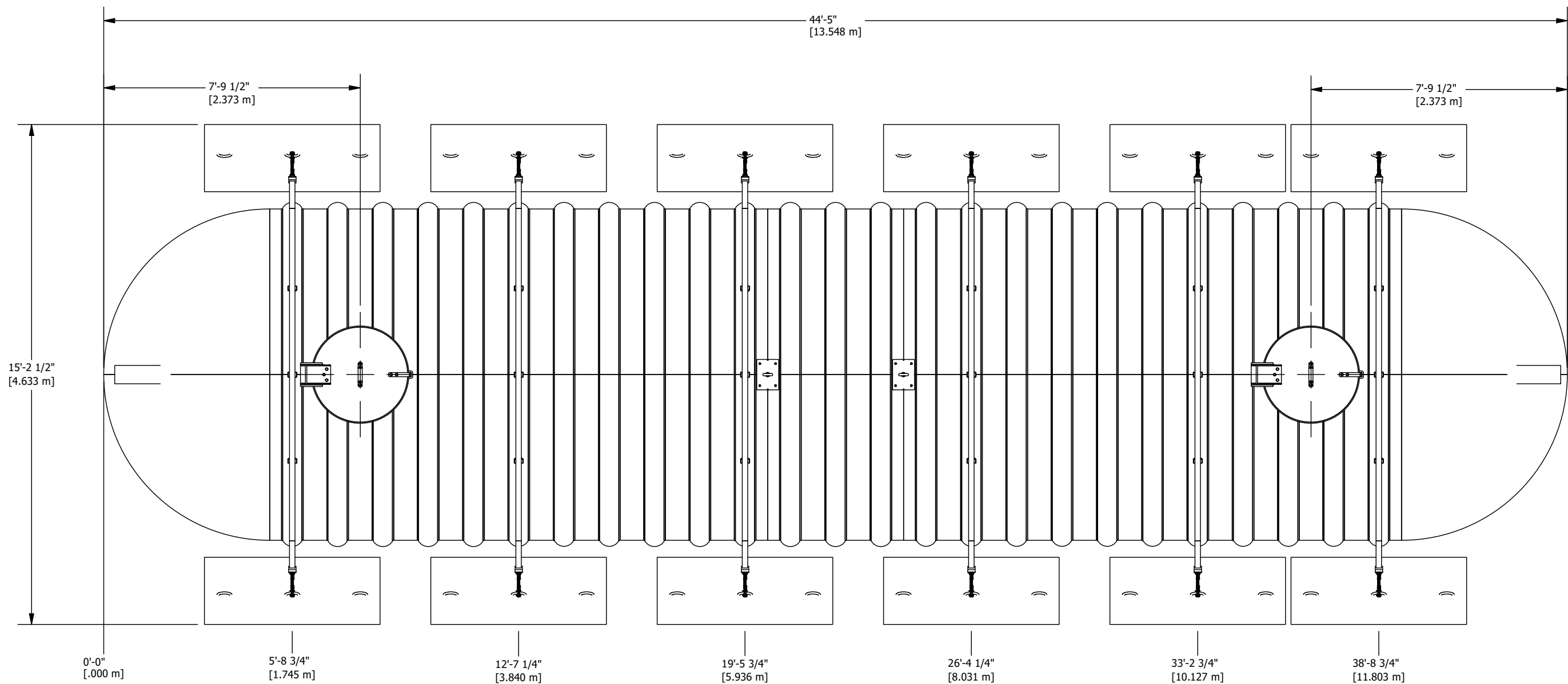
VUE DE PLAN PLAN VIEW
