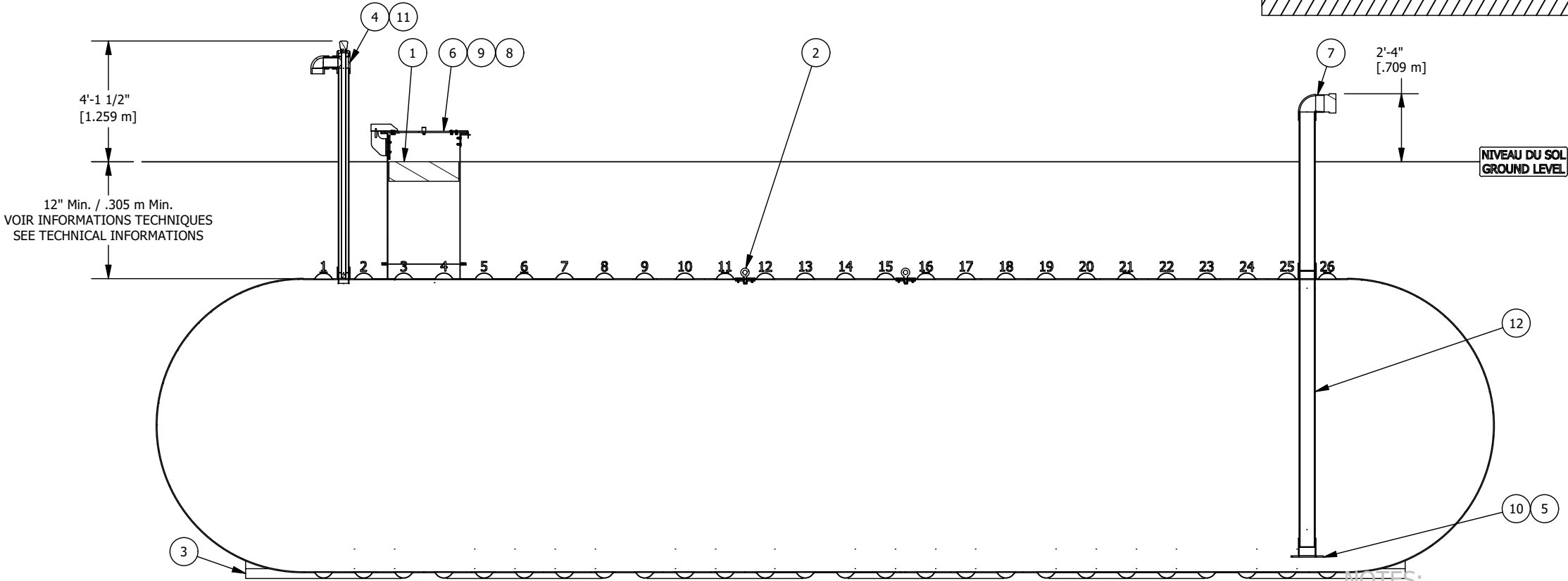
VUE D'ÉLEVATION COUPÉE CUT ELEVATION VIEW
