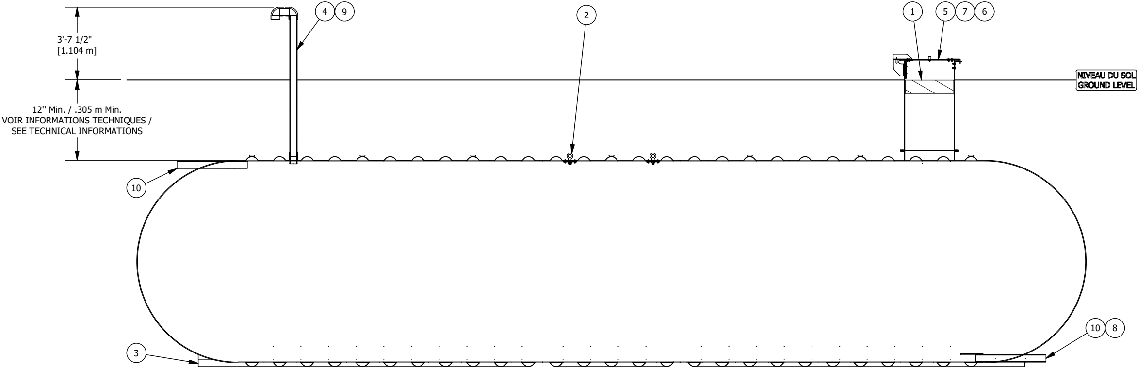
VUE D'ÉLEVATION COUPÉE CUT ELEVATION VIEW
