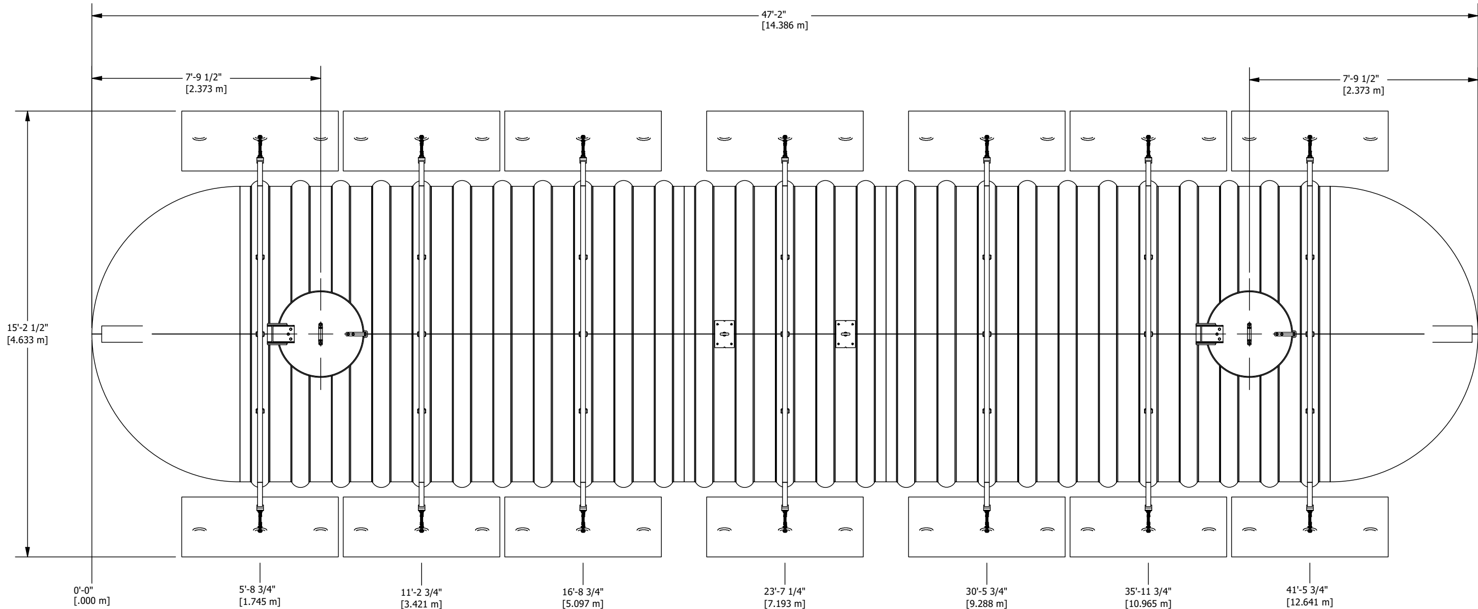
VUE DE PLAN PLAN VIEW
