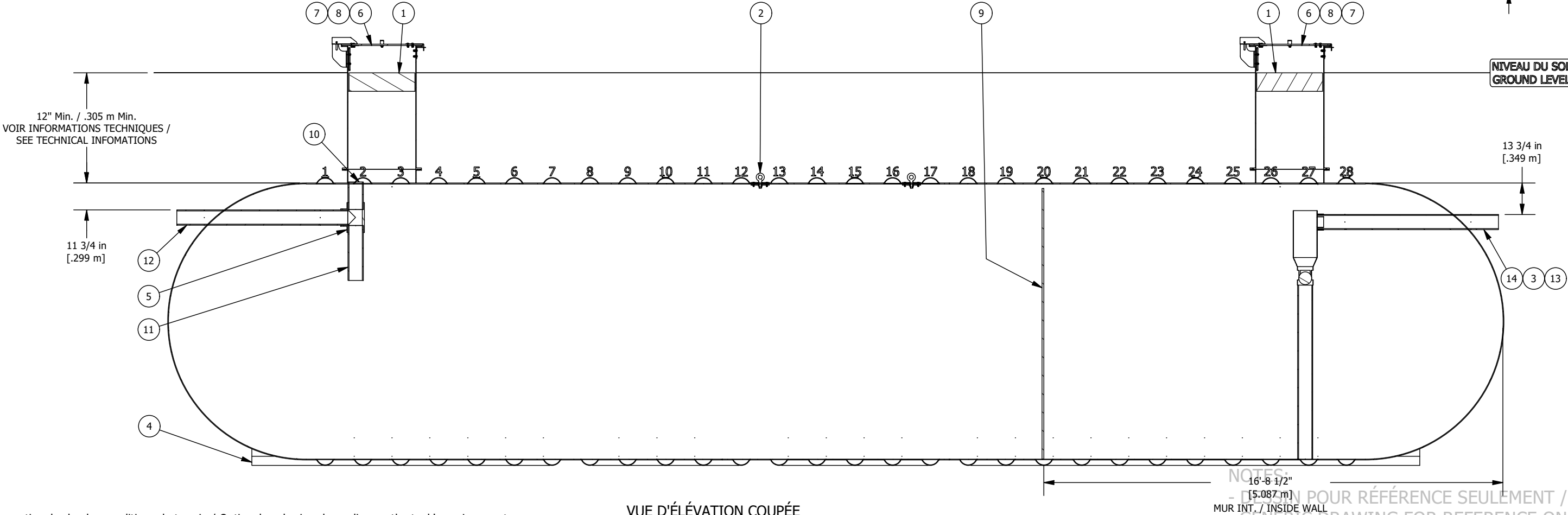
VUE D'ÉLEVATION COUPÉE CUT ELEVATION VIEW
