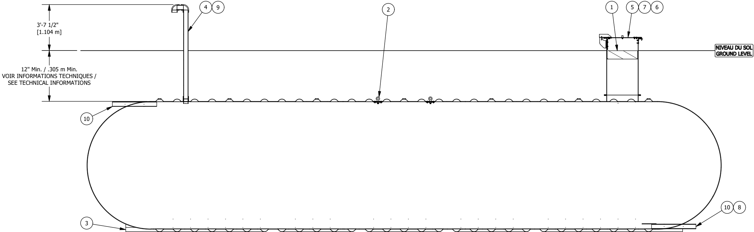
VUE D'ÉLEVATION COUPÉE CUT ELEVATION VIEW
