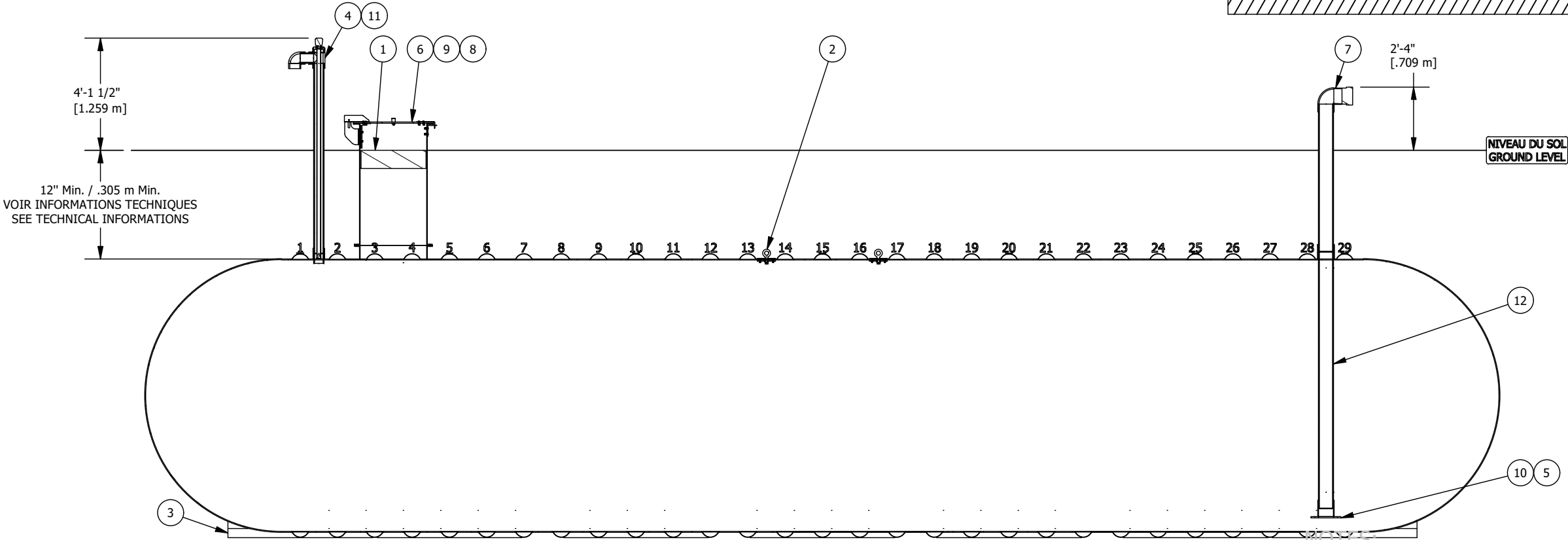
VUE D'ÉLEVATION COUPÉE CUT ELEVATION VIEW
