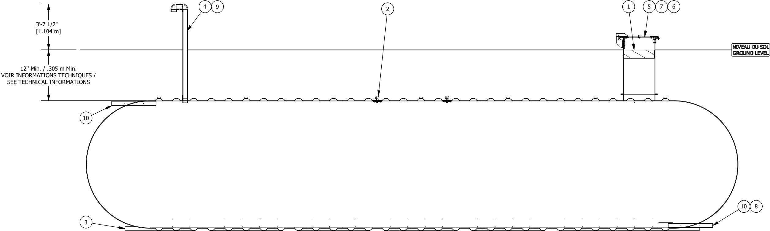
VUE D'ÉLEVATION COUPÉE CUT ELEVATION VIEW
