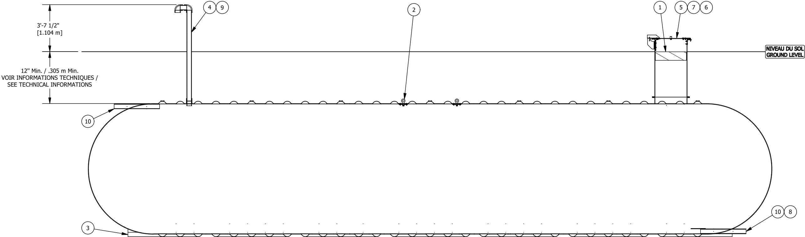
VUE D'ÉLEVATION COUPÉE CUT ELEVATION VIEW
