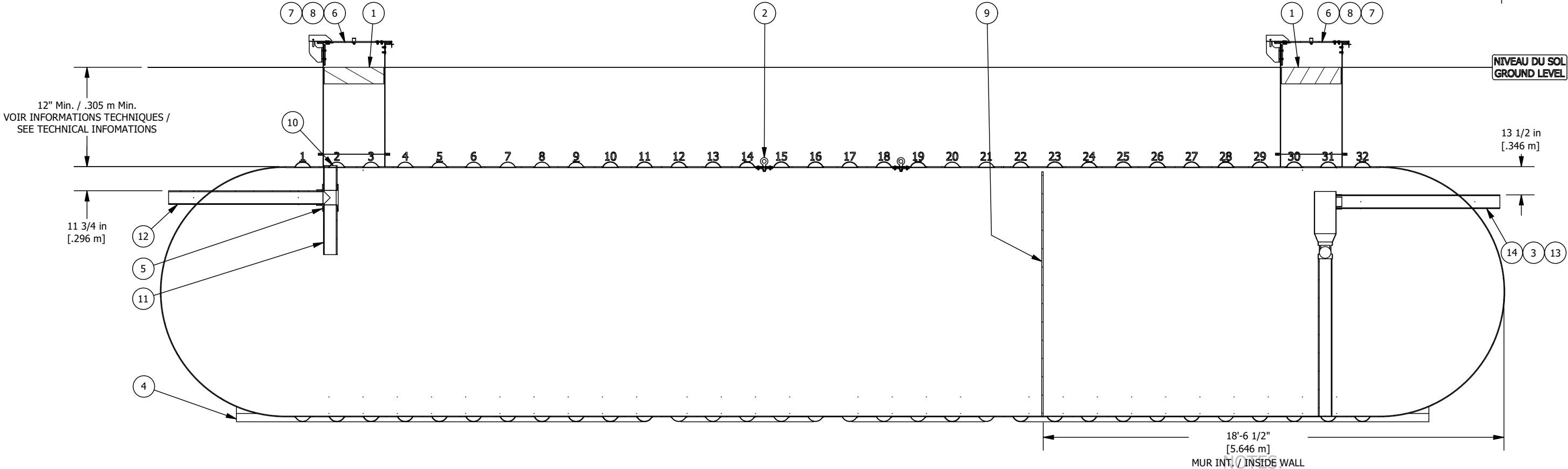
VUE D'ÉLEVATION COUPÉE CUT ELEVATION VIEW
