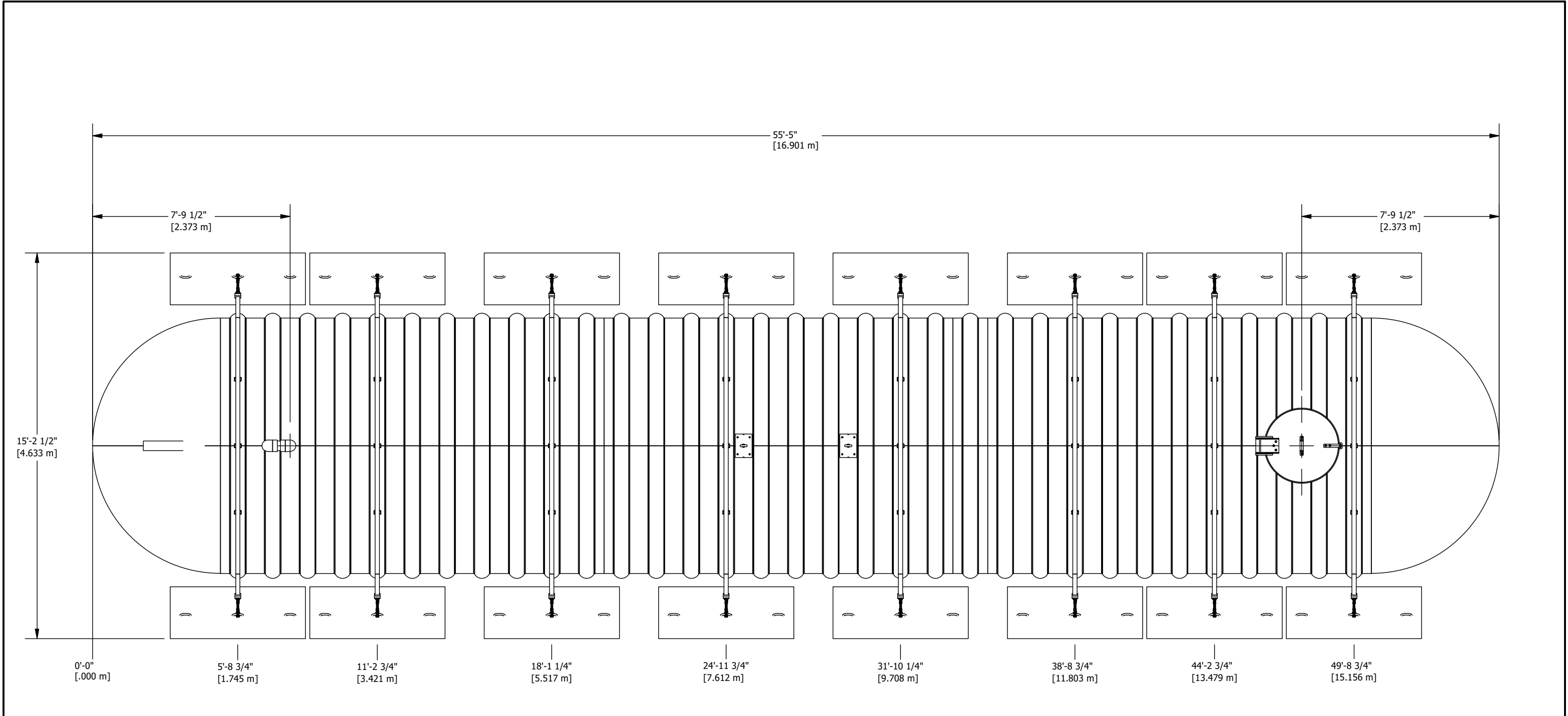
VUE DE PLAN PLAN VIEW
