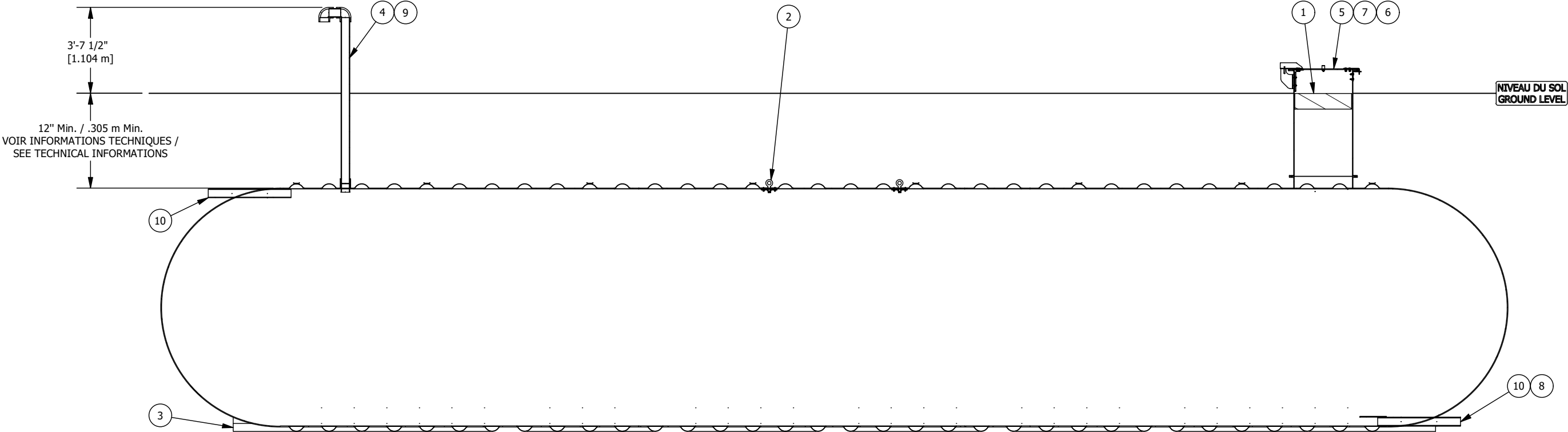
VUE D'ÉLEVATION COUPÉE CUT ELEVATION VIEW
