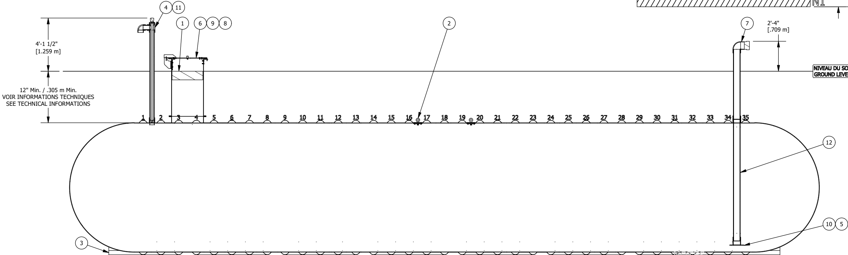
VUE D'ÉLEVATION COUPÉE CUT ELEVATION VIEW
