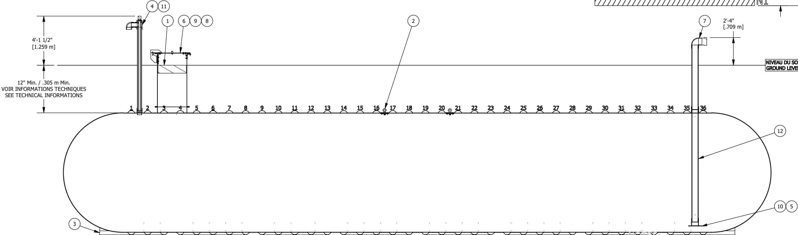
VUE D'ÉLEVATION COUPÉE CUT ELEVATION VIEW
