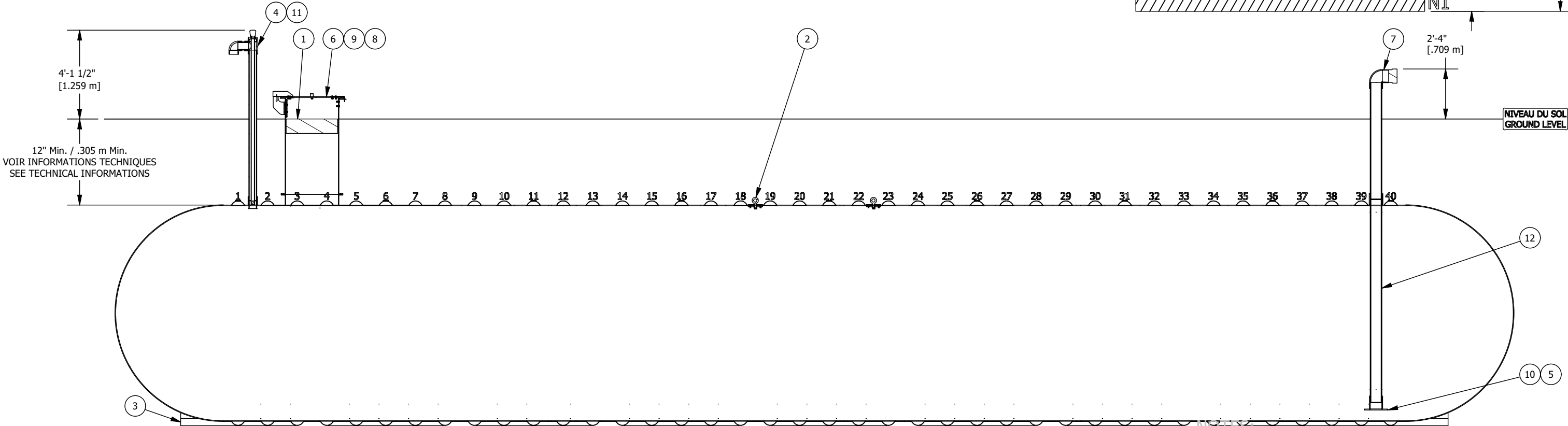
VUE D'ÉLEVATION COUPÉE CUT ELEVATION VIEW
